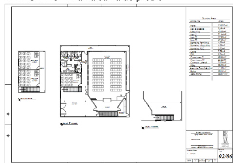
IMAGEM 3 – Planta baixa do prédio
